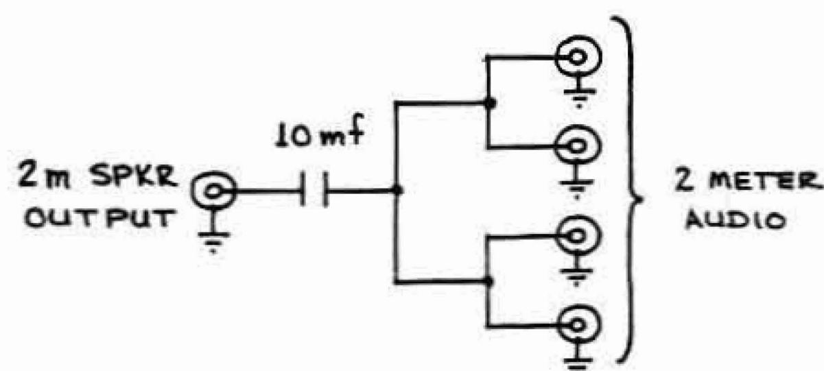
2 METER SPLITTER
